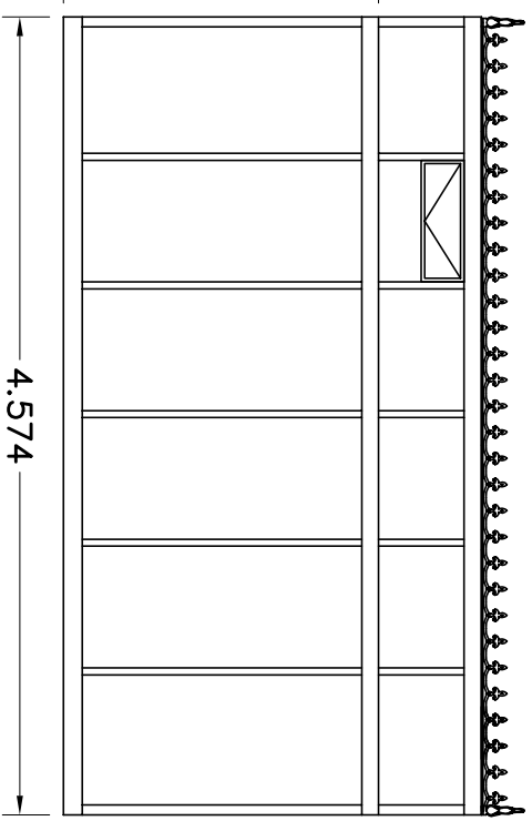
AANZICHT B
