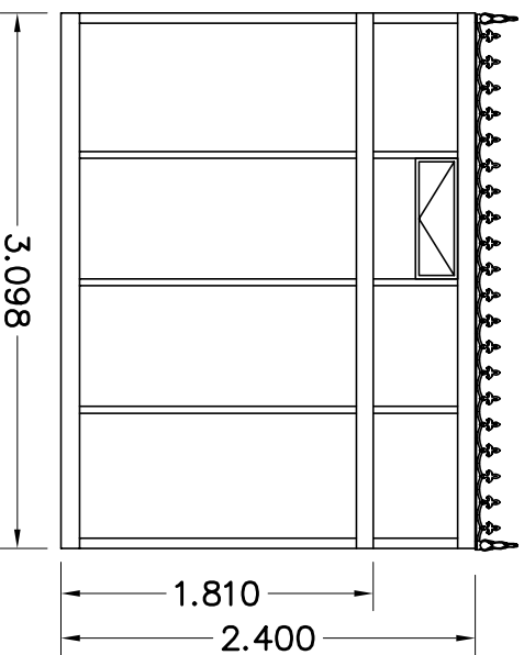
AANZICHT D
