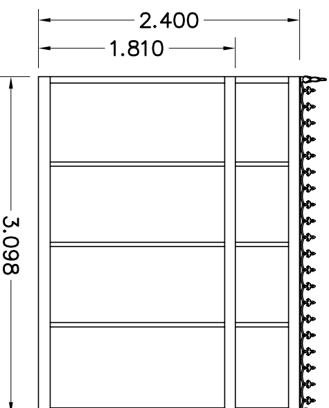
AANZICHT B
