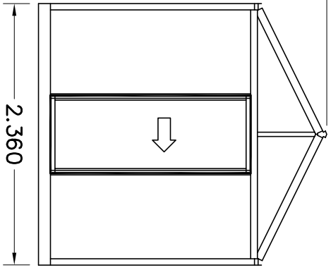
AANZICHT A
