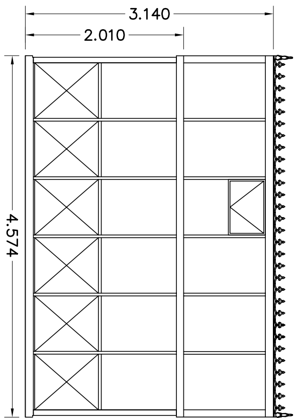
AANZICHT D
