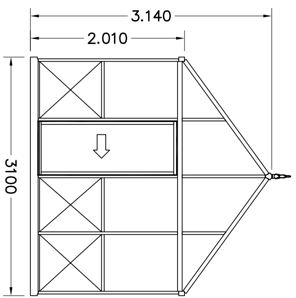
AANZICHT A
