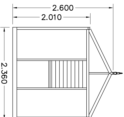
AANZICHT C
