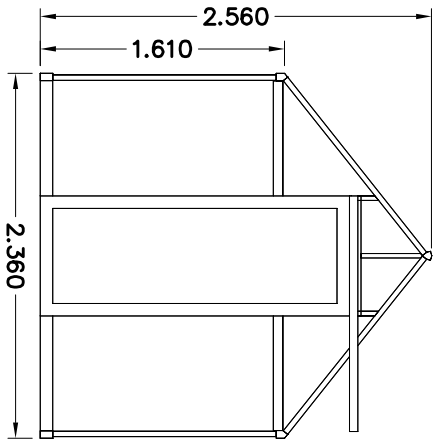
AANZICHT A
