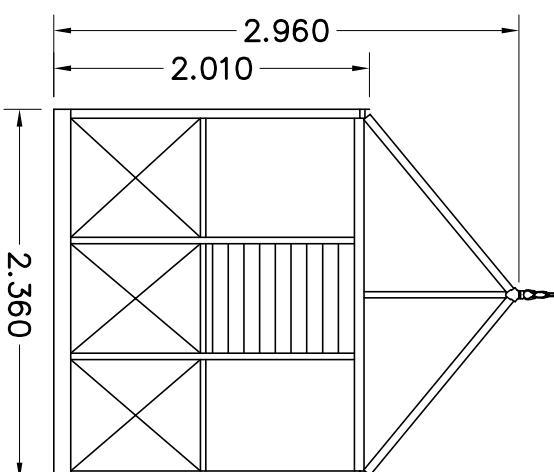
AANZICHT C
