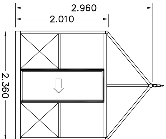
AANZICHT A
