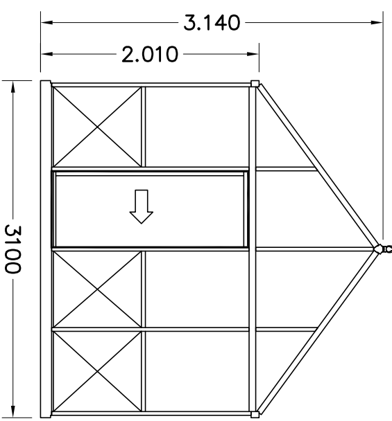
AANZICHT C
