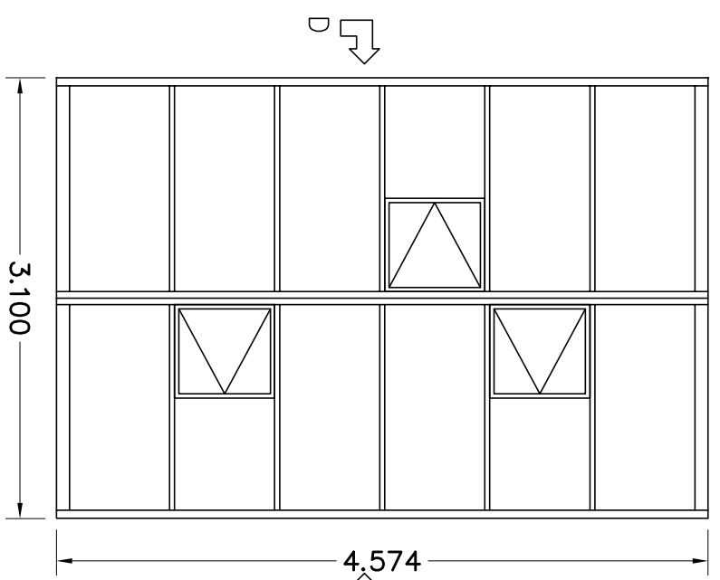
BOVENAANZICHT ↻ C
