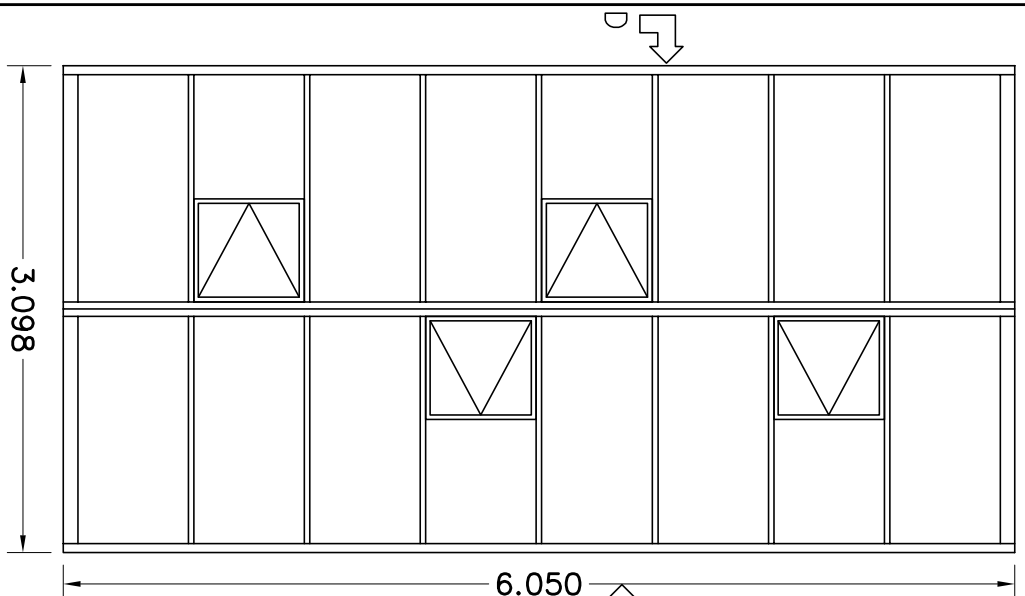
BOVENAANZICHT ↻ C
