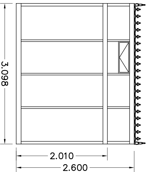
AANZICHT D
