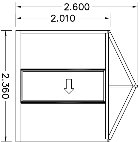
AANZICHT A
