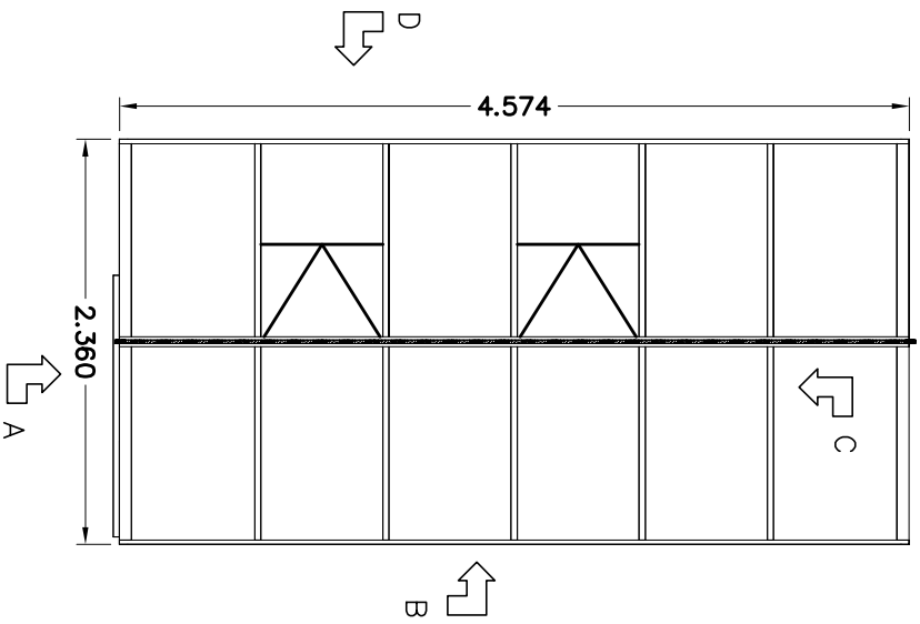
BOVENAANZICHT
