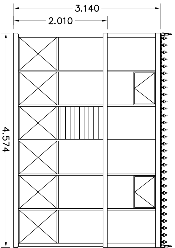
AANZICHT B
