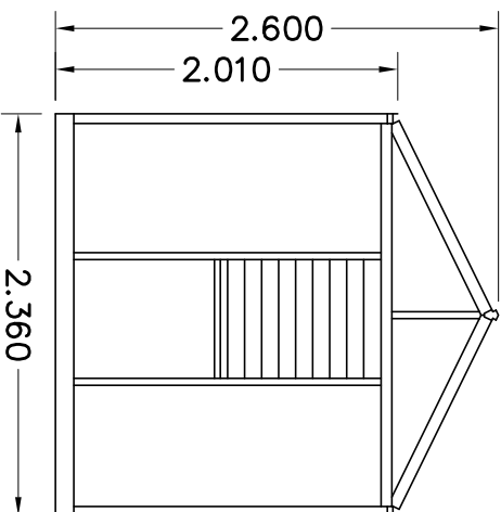
AANZICHT C
