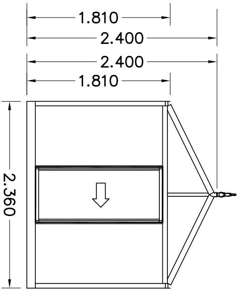
AANZICHT A
