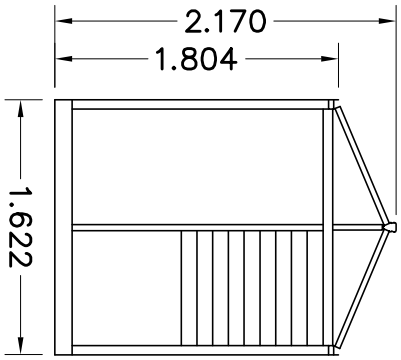
AANZICHT A
