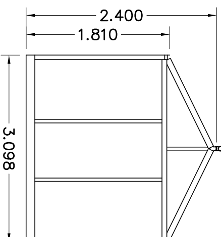
AANZICHT C
