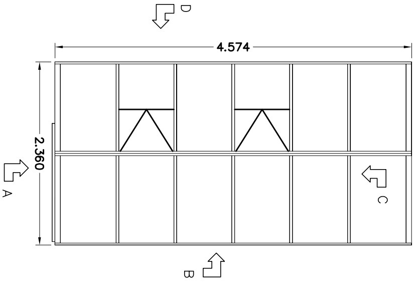
BOVENAANZICHT
