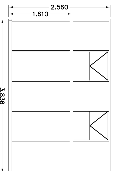
AANZICHT D
