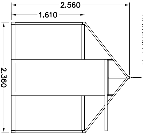
AANZICHT A
