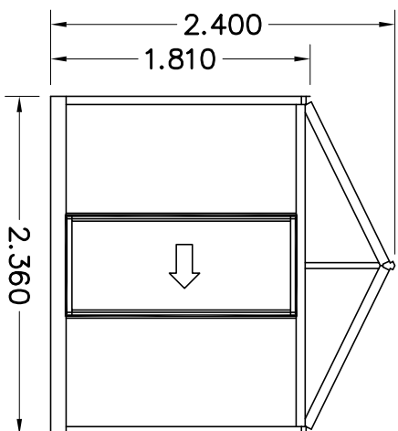
AANZICHT A
