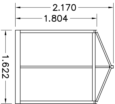
AANZICHT C
