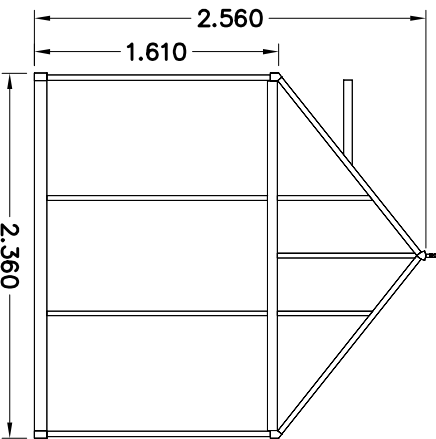
AANZICHT C
