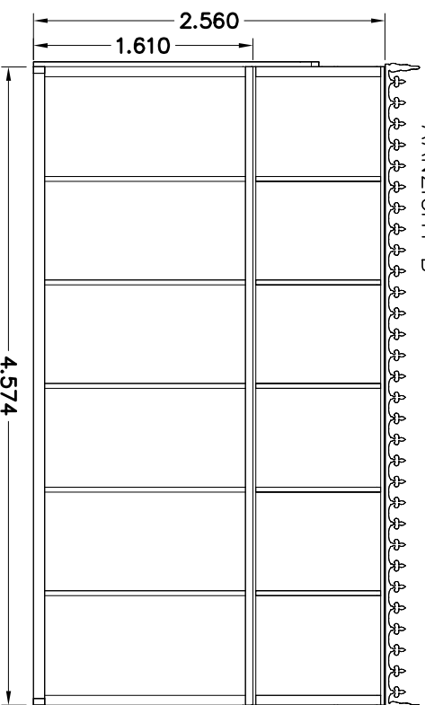
AANZICHT B
